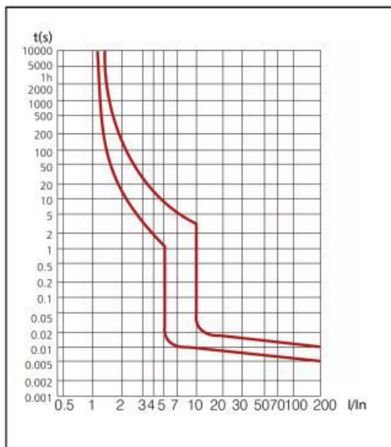
Kennlinie C
