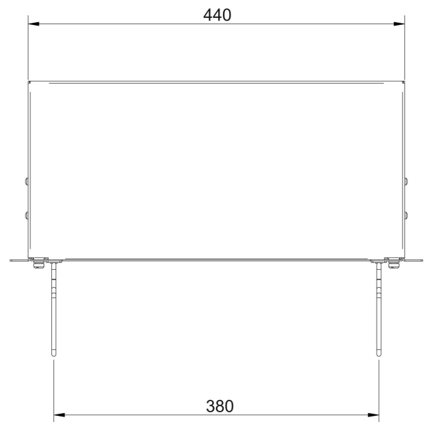
Draufsicht
