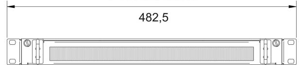
Frontansicht
