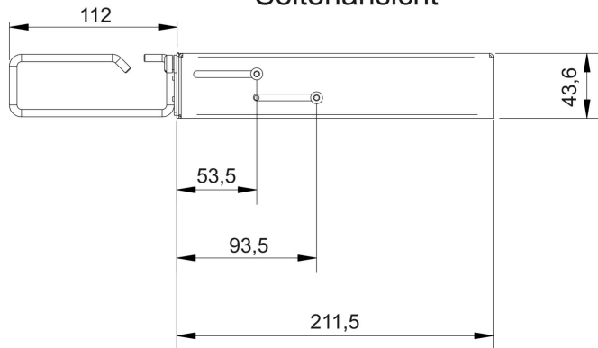
Seitenansicht
